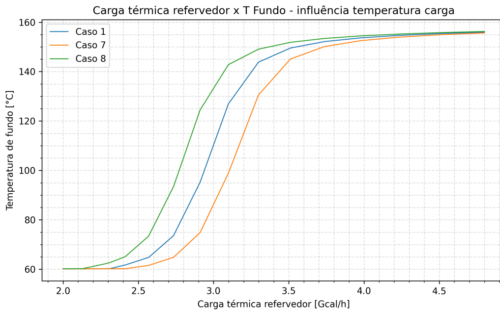
Figura 8: Carga térmica x temperatura do fundo - Influência da temperatura da carga
